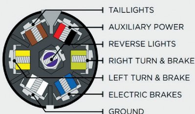
7 RV (SAE)
