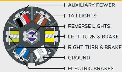
7 RV (SAE)
